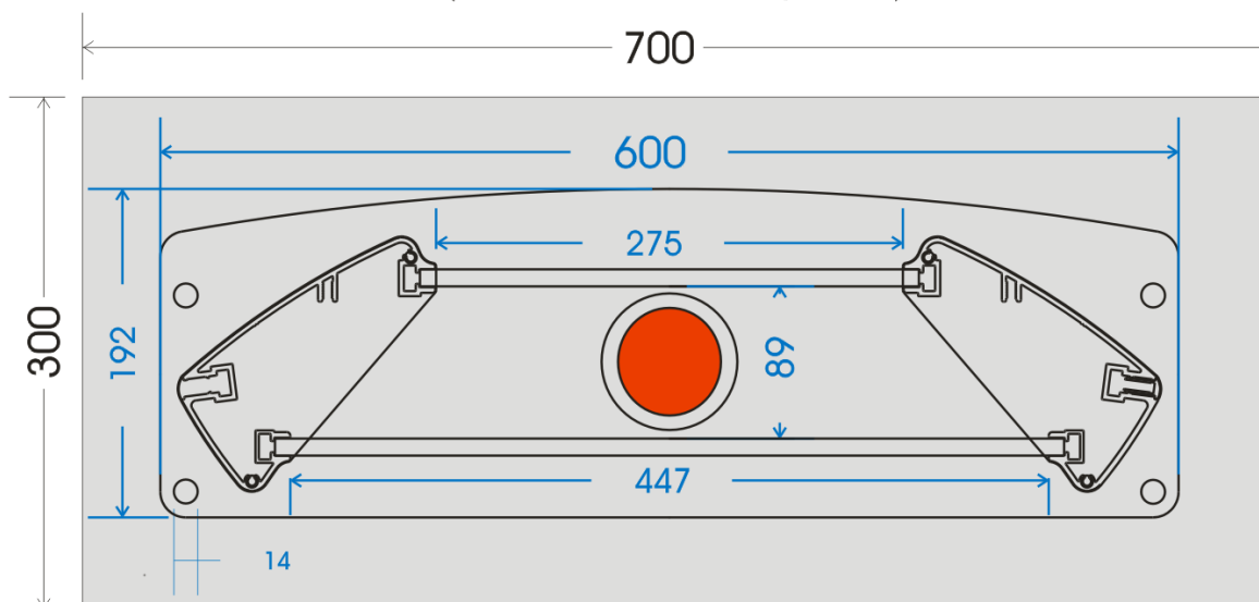
Massif béton dosé à 350 Kg/m 3 700/300/500 L x l x Pr avec fourreau de 63 dans l'axe
