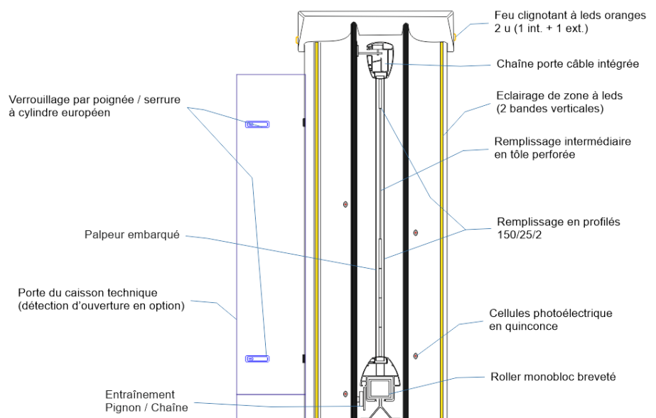
COUPE PORTAIL ULMALU® 800 RAPID
